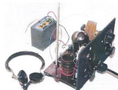
▲ Собранный в ТИИ по схеме, аналогичной Косухинской, портативный радиоприемник
