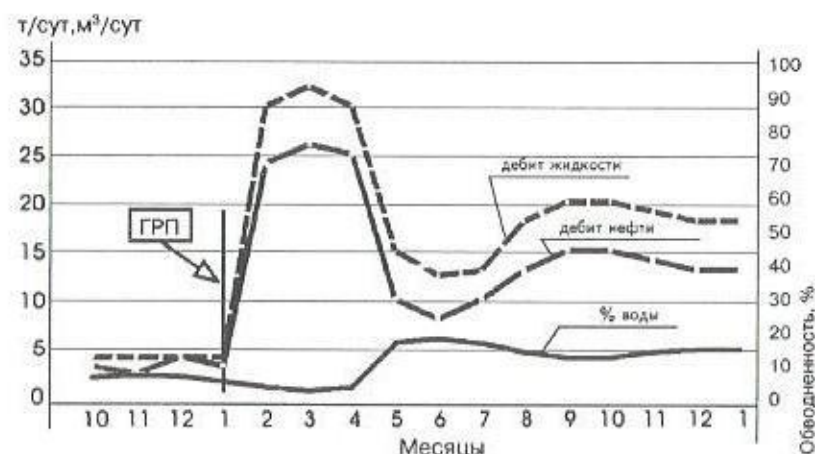
Рис. 31. Динамика работы скважин после ГГРП
